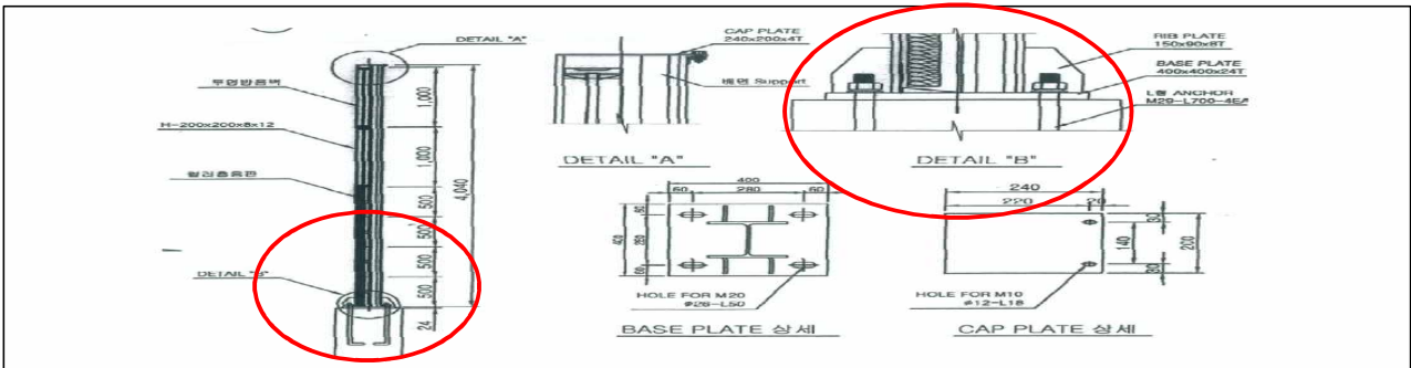
[그림 1] (당초 설계) 방음벽 지주 시공방법 현황도
