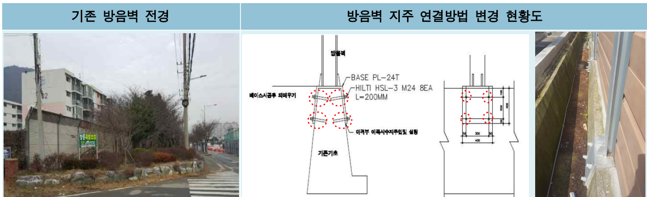
[그림 2] 방음벽 지주 설계변경 현황도
